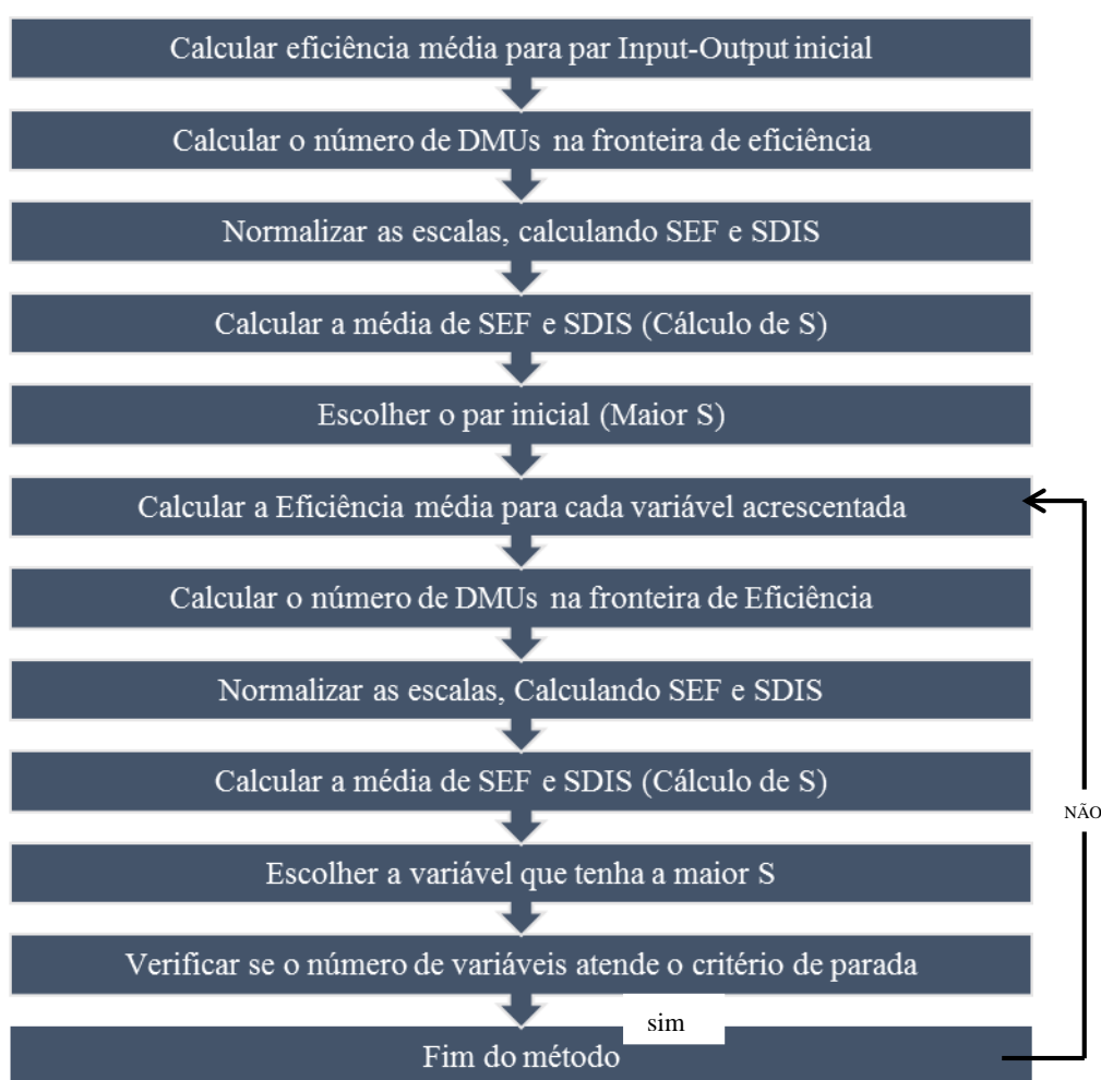
Figura 2: Método Combinatório Multicritério Inicial
